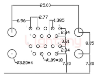
PCB布局 (PCB Layout)
