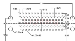
PCB布局 (PCB Layout)
